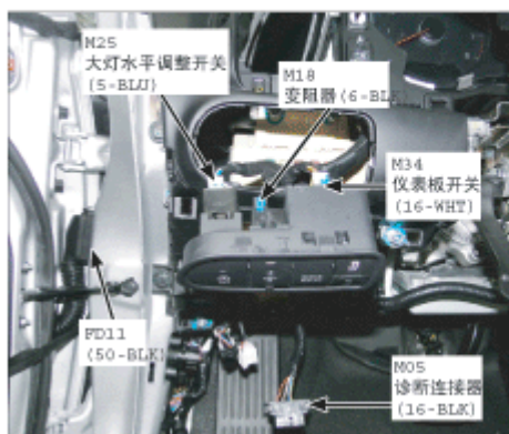
40. 仪表板左侧
